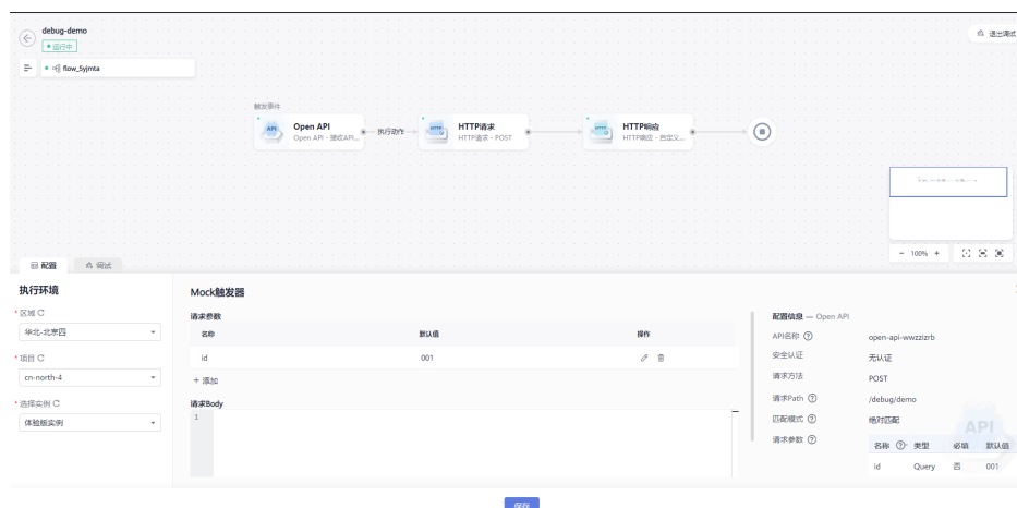
图 5-2 调试窗口
