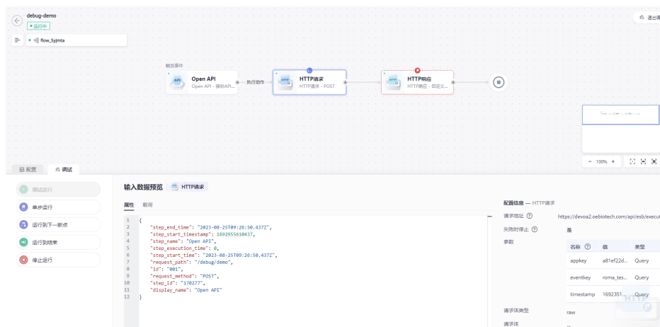
图 5-6 单步调试
